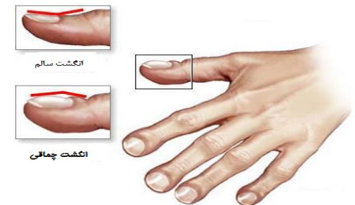
شکل ۱: انگشتان چماقی
